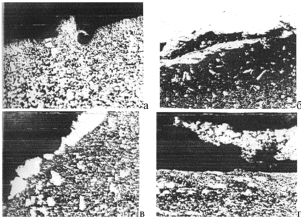
Рисунок 5 – Мікрофотографії (x200) поверхонь пуансонів зі сталі У8А, які працювали в умовах пошкоджуваності: а – задири на пуансоні; б – схоплювання; в – налипання металу заготовки; г – розпушення поверхневого шару пуансона
