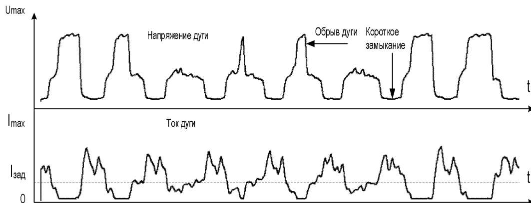
Рисунок 1 – Скачкообразное изменение тока дуги в процессе обработки детали
