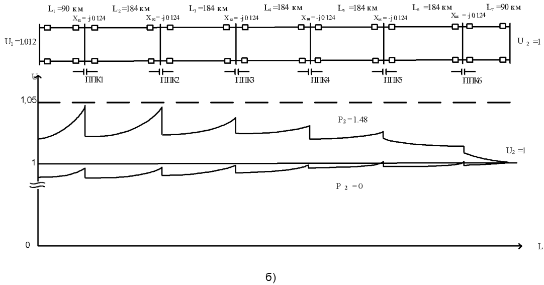
Рисунок 1 – Розподіл напруги вздовж лінії
