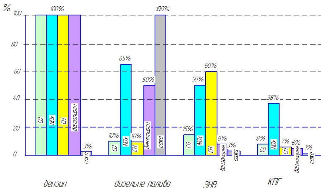
Рис. 1. Порівняння екологічних показників різних видів палив
