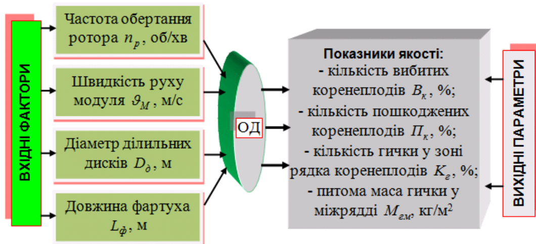
Рис. 2. Загальна схема структурної моделі комбінованого копача
