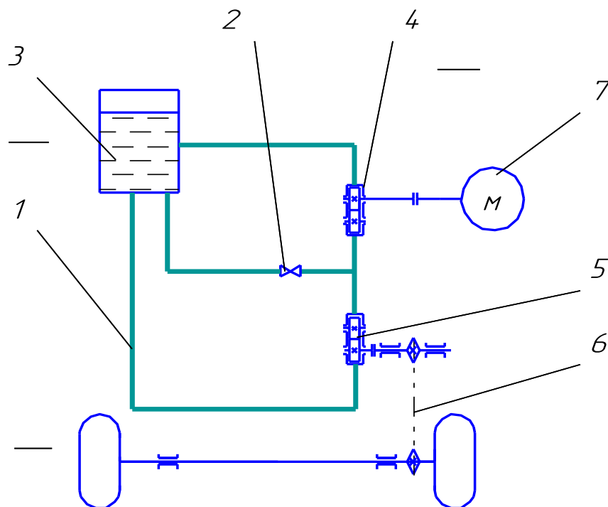
Рис. 1. Схема удосконаленого механізму передач:
