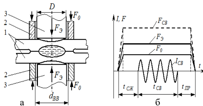
Рис. 1. Схема (а) та цикл зміни параметрів режиму (б) двостороннього КТЗ з обтисненням периферійної зони з'єднання:
