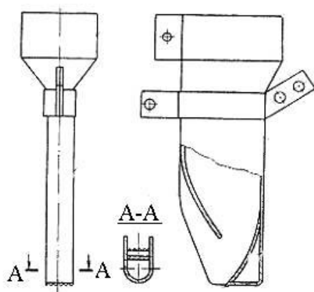
Рис.1. Універсальний наральниковий сошник
