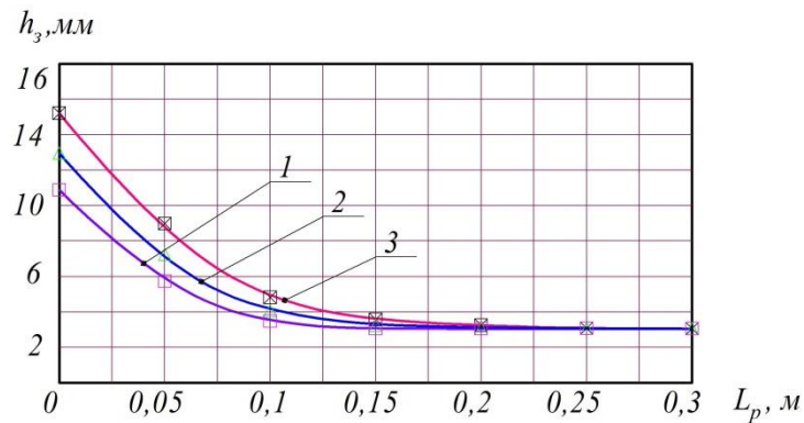
Рис. 2. Залежність зміни товщини шару зернового потоку h_z по довжині розгінної ділянки прямої кривої живильника L_p при \alpha = 36^\circ : 1 – q_B = 250 кг/дм·год; 2 – q_B = 350 кг/дм·год; 3 – q_B = 500 кг/дм·год;
