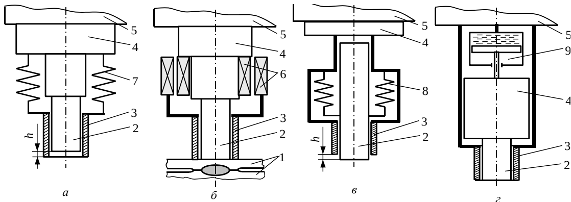
Рис. 2. Електродні пристрої для КТЗ з обтисненням периферійної зони з'єднання:
