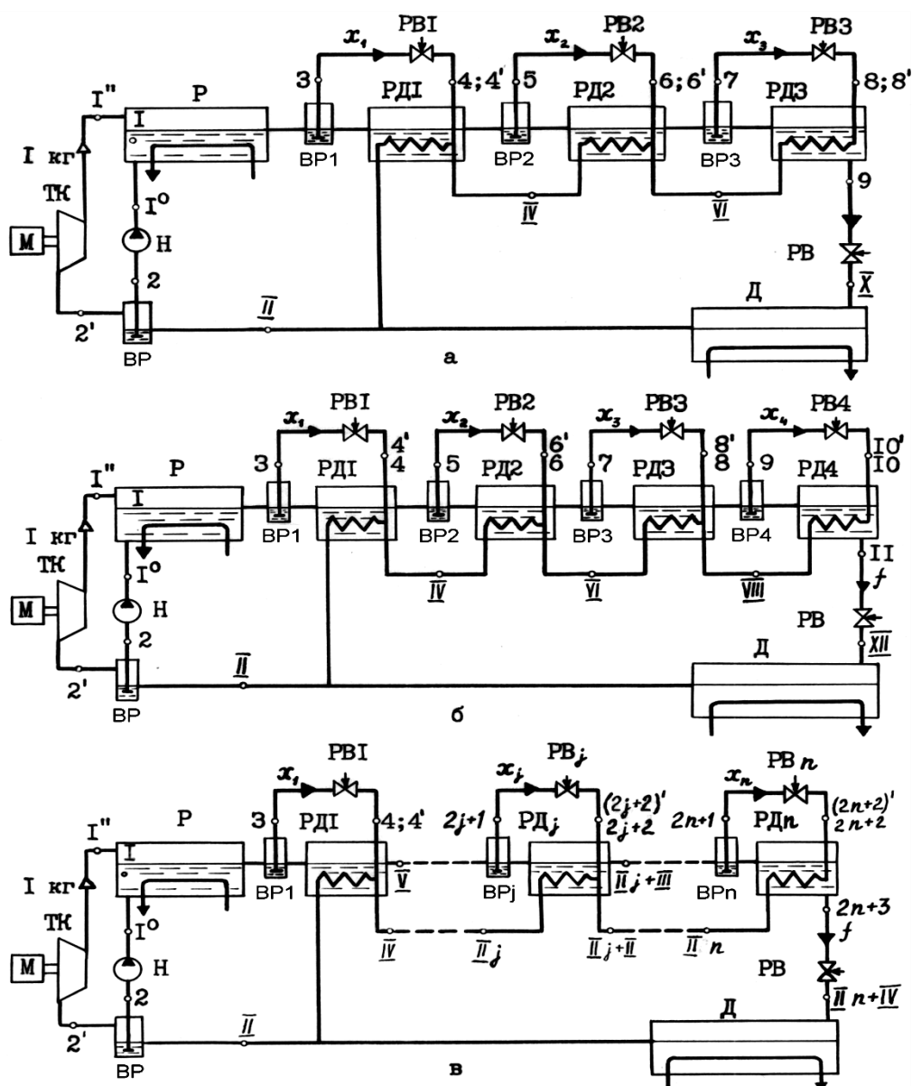
Рис. 1. Схеми КРХМ:
