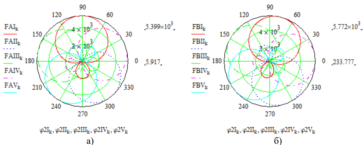
Рис. 2. Годографы реакций F_A (а) и F_B (б) в Н на опорах соломотряса
