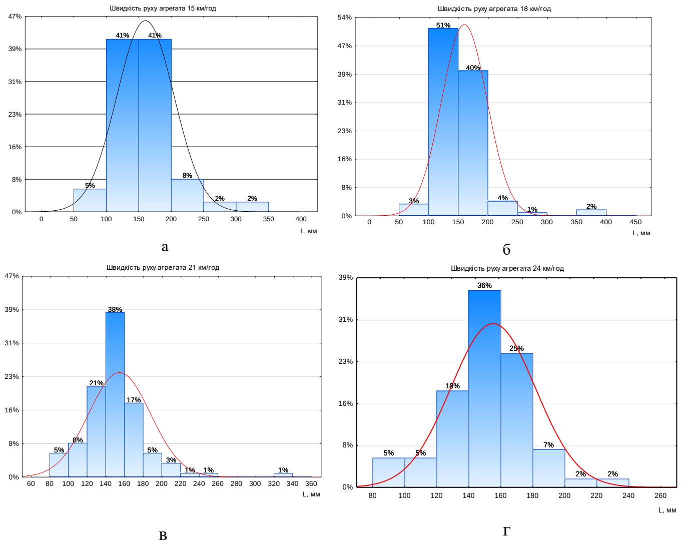
Рис. 2. Гістограма розподілу решток стебел кукурудзи за довжиною L після обробітку при різних швидкостях руху агрегату: а– ступінь подрібнення C=88\% при швидкості 15 км/год; б– ступінь подрібнення C=93\% при швидкості 18 км/год; в– ступінь подрібнення C=94\% при швидкості 21 км/год; г– ступінь подрібнення C=96\% при швидкості 24 км/год.
