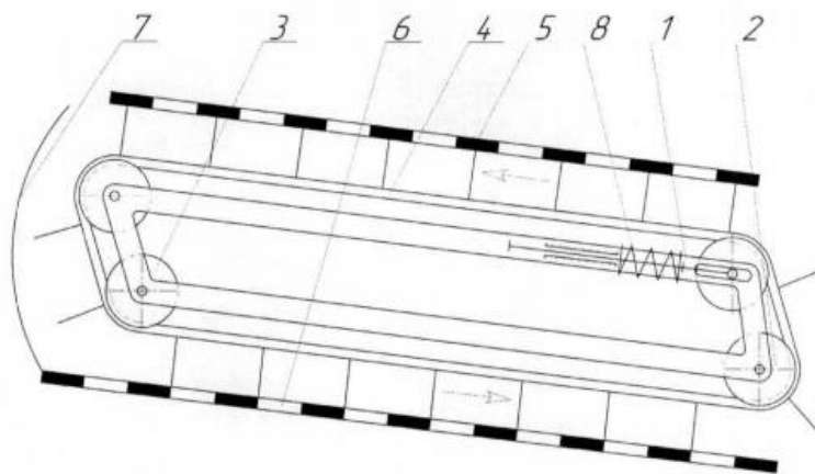
Рис. 2. Схема удосконаленого очисного пристрою
