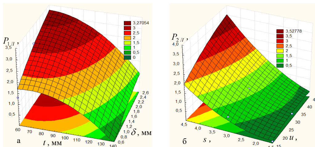
Рис. 2. Поверхня відгуку зміни зусилля стиснення електродів P_{1d} як функція P_{1d} = f_1(t, \delta)
