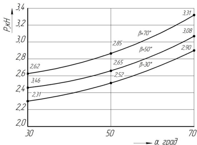
Рис. 2. Залежність опору різання від кутів постановки диска до напрямку руху ( \alpha ) і вертикалі ( \beta ), чорнозем, глибина ходу 25 см
