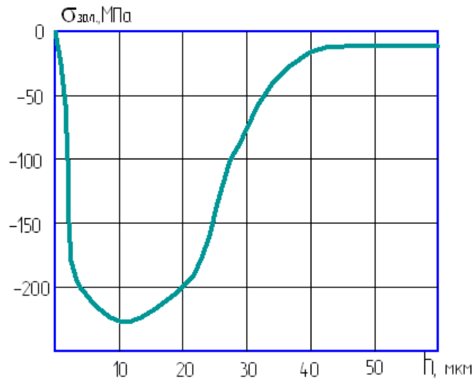
Рис. 2. Розподіл залишкових напружень по глибині азотованого шару.
