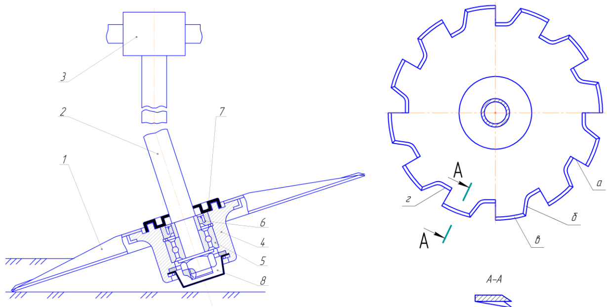
Рис 1. Дисковий ґрунтообробний робочий орган
