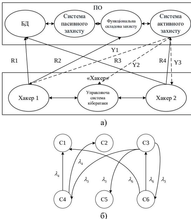
Рис. 1. Структурна схема способу оцінки ефективності методу підвищення безпеки ПЗ та розмічений граф станів системи
