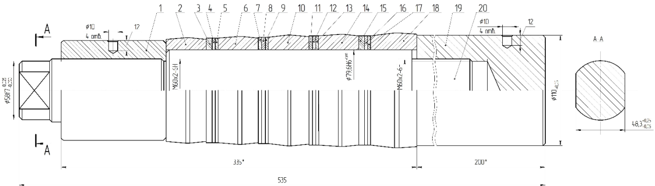
Рисунок 1 – Деформуюча протяжка
