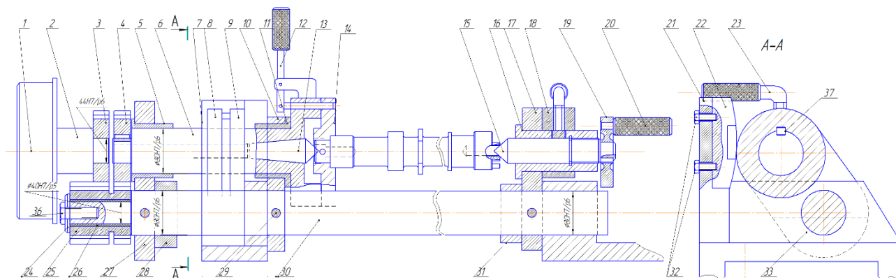
Рисунок 1. Загальний вигляд пристосування (позначення в тексті)
