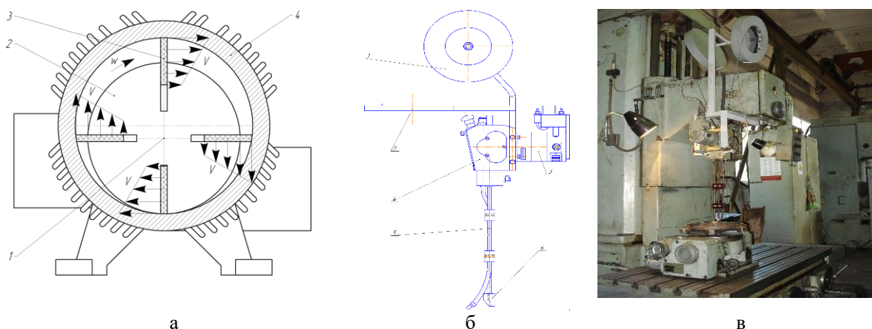
Рисунок 1 -Технологічні особливості відновлення корпусів компресора: а) корпус насоса в розрізі та схема дії сил: 1 – вісь ротора; 2 – ротор; 3 – пластина; 4 – корпус; б) електродуговий розпилювач: 1 - касети з дротами, 2 – фланець кріплення, 3 – електродвигун постійного струму, 4 – корпус редуктора; 5 – направляючі для ПД, 6 – сопло розпилювача; в); компоновка технологічного обладнання.
