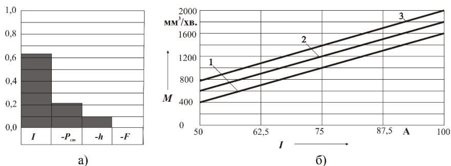
Рисунок 1 – Продуктивність M бічної поверхні зразка з використанням способу зворотного прокачування (а - ступінь впливу змінних факторів; б - залежність M від I ; 1 - P_{cm} = 1,2 МПа; 2 - P_{cm} = 1,0 МПа; 3 - P_{cm} = 0,8 МПа
