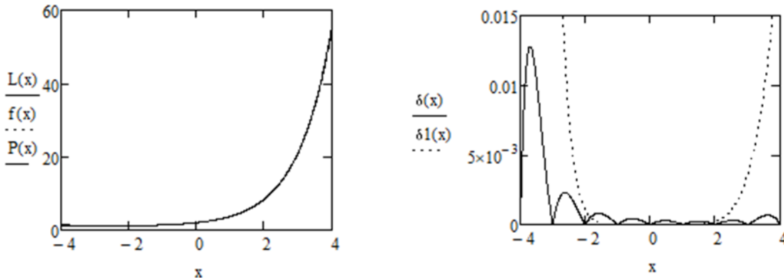
Рисунок 2 – Графік функції f(x) = e^x + 1 та її наближення многочленами (зліва); графік відносних похибок (справа)
