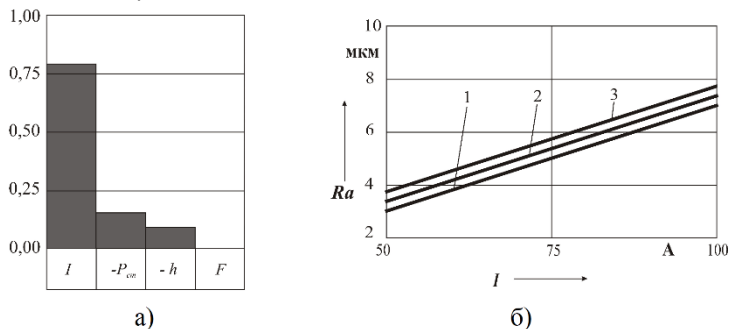
Рисунок 2 – Шорсткість Ra обробленої поверхні з використанням способу зворотного прокачування (а - ступінь впливу змінних факторів; б - залежність Ra від I ; 1 - P_{cm} = 1,2 МПа; 2 - P_{cm} = 1,0 МПа; 3 - P_{cm} = 0,8 МПа)
