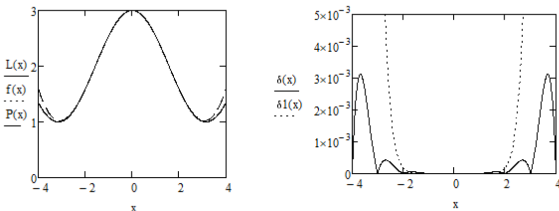
Рисунок 1 – Графік функції f(x) = \cos(x) + 2 та її наближення многочленами (зліва); графік відносних похибок (справа)
