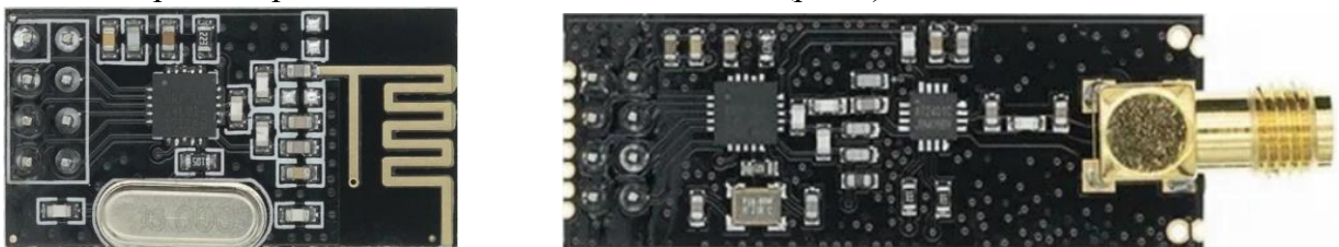
Рисунок 1 - Трансивери NRF24L01+ та NRF24L01+PA+LNA
